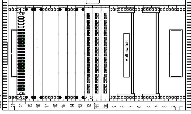
Szafa wisząca dwuczęściowa, BKT TOP 21U, 600/600, RAL 7035 11049001.1.V
